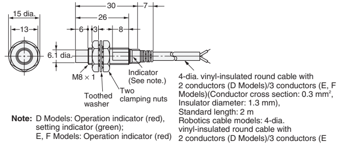
Fig. 5 : E2E-X4MD□ E2E-X2ME□/F□
