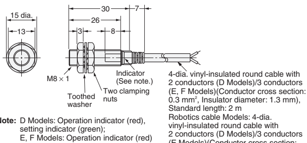
Fig. 4 : E2E-X2D□-N E2E-X1R5E□/F□
