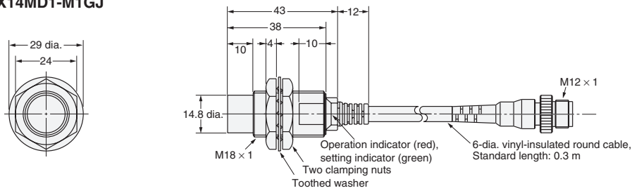
Fig. 32 : E2E-X14MD1-M1GJ
