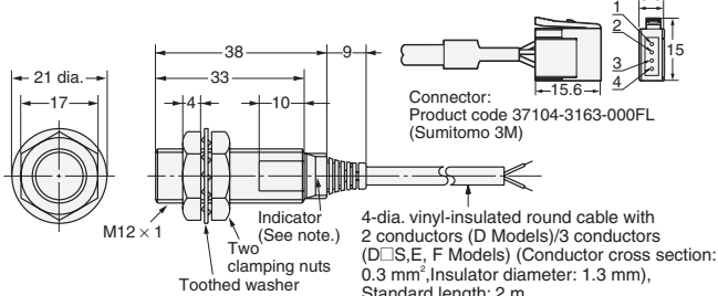
Fig. 8 : E2E-X3D□-N E2E-X2E□/F□
