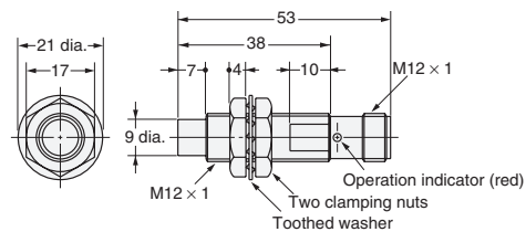
Fig. 24 : E2E-X14MD□-M1(G)/E2E-X10ME□-M1/F□-M1 E2E-X10MY□-M1
