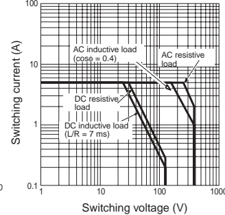
G2R-2-S
