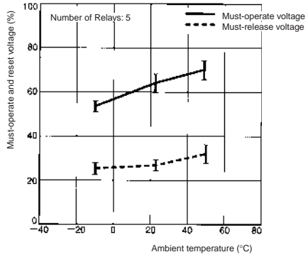
G7J 24 VDC
