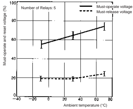
G7J 24 VDC
