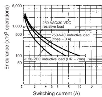
G2R-1-S
