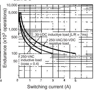
G2R-2-S
