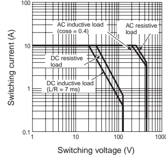
G2R-1-S
